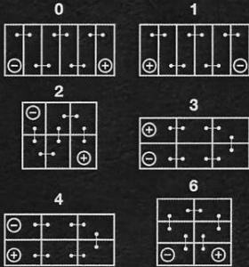
Esquema 12 V
